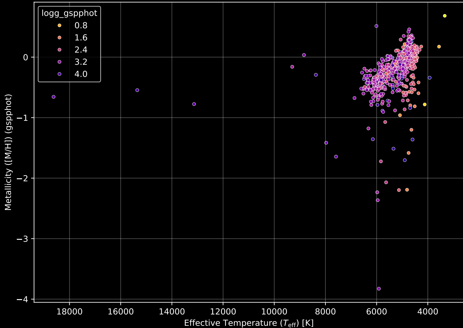
APOGEE DR17 Field: [M22] Stellar Population Parameters (n= 607)
